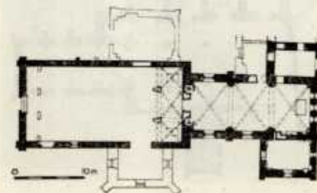
9. Plan kościoła franciszkanów w Zawichocinie
