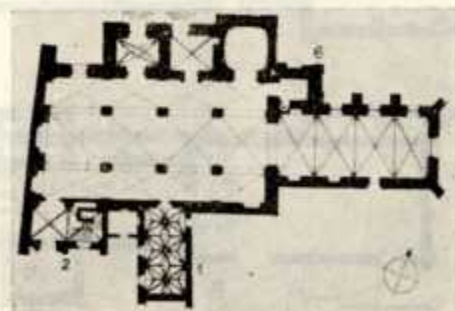
12. Plan kościoła franciszkanów w Opolu
